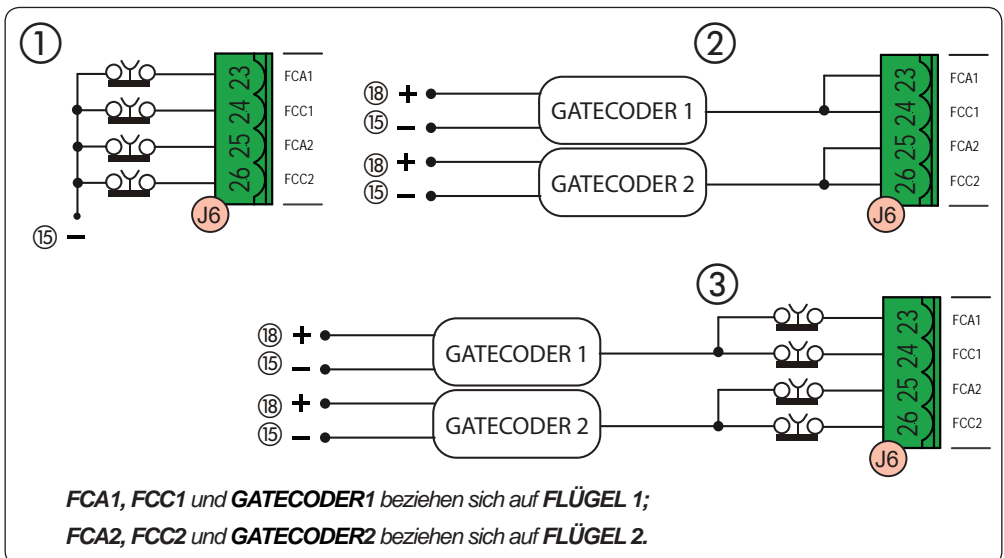
Abb. Anschlüsse Endschalter und GATECODER (maximale Konfiguration: ③).
