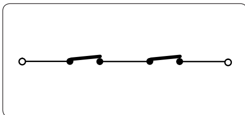
Abb. Reihenschaltung von zwei Öffnerkontakten
